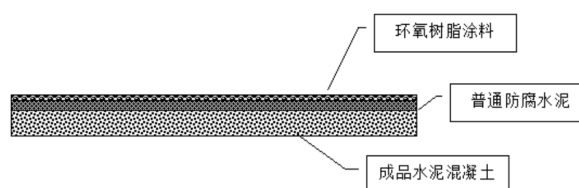
图 4-5 重点区域防渗层剖面图
