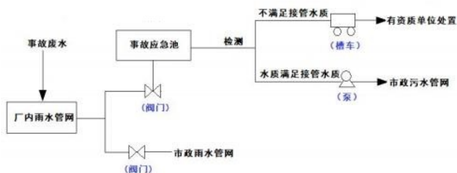
图 4-6 事故排水控制和封堵示意图
