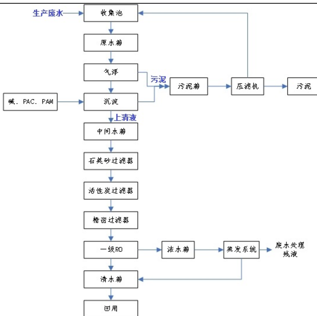
图 4-3 污水处理设施工艺流程图
